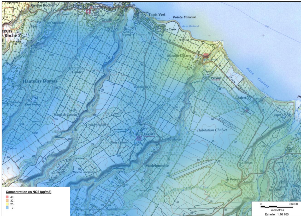
IV.4 Spatialisation de la pollution automobile sur la commune de Basse-Pointe, moyennée sur les 4 campagnes de mesure.
