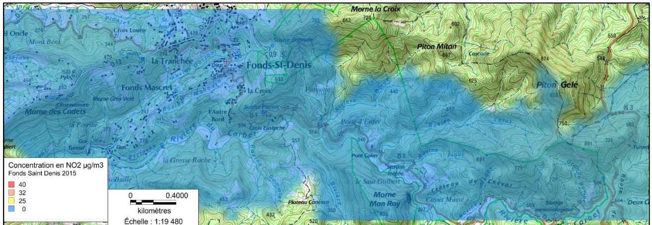
Figure IV-4 : Spatialisation de la pollution automobile sur la commune de Fonds Saint Denis, moyennée sur les 4 campagnes de mesure.
