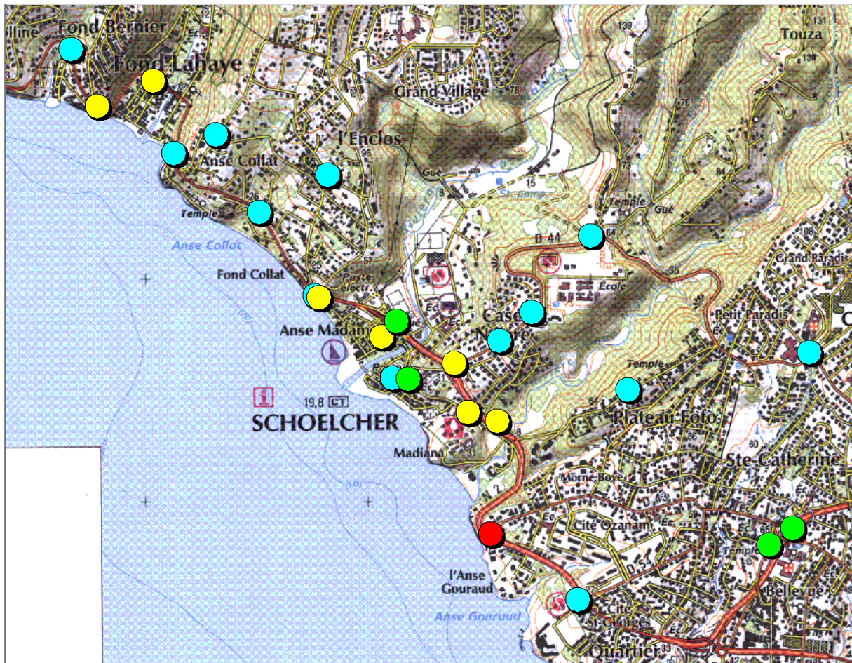
Annexe VI.3 : Dispersion de la concentration en NO 2 ( \mu\text{g}/\text{m}^3 ) sur la commune de Schœlcher durant la Campagne 2 du 29/09/2008 au 13/10/2008.
