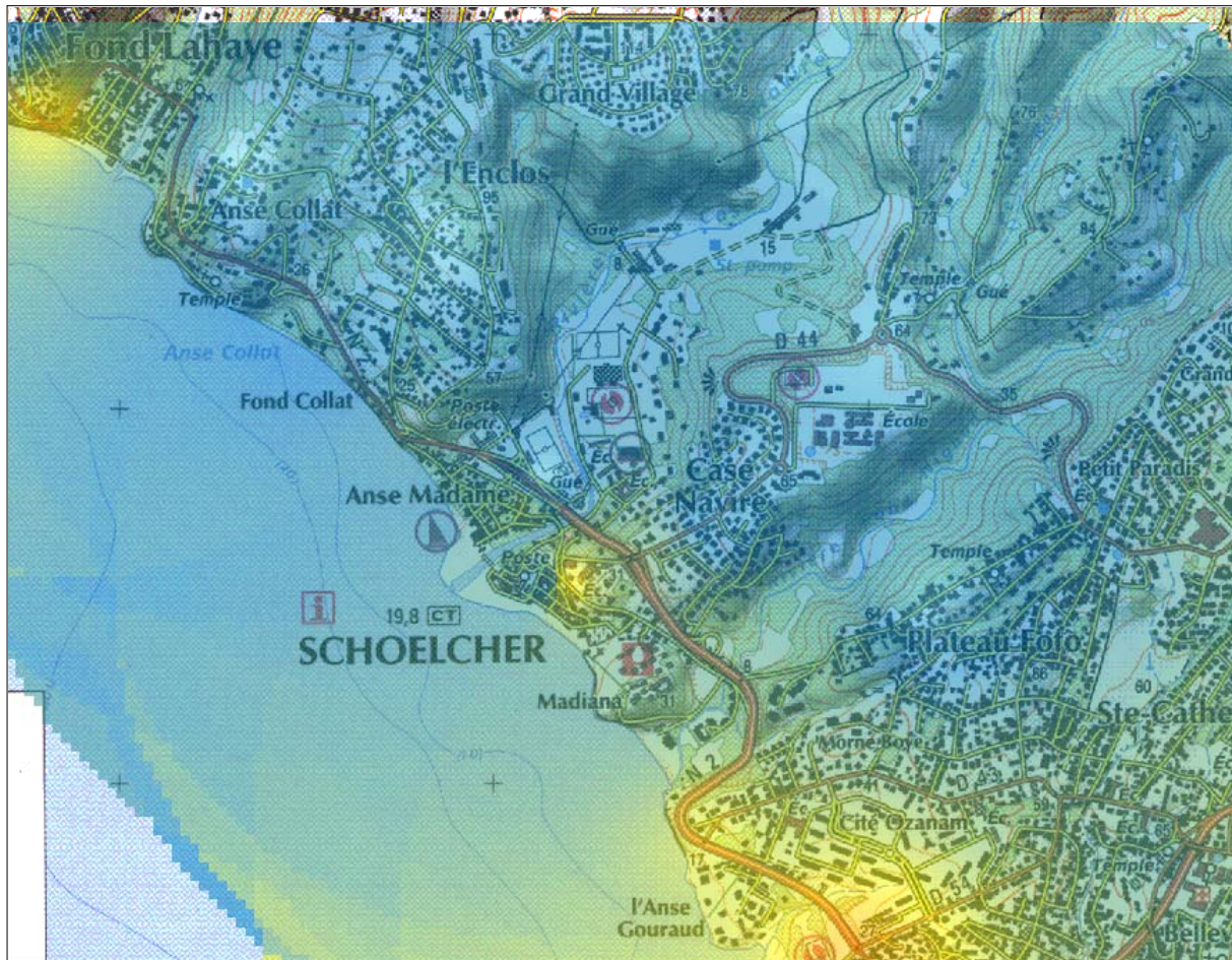
Annexe VI.6 : Dispersion de la concentration moyenne en NO 2 (µg/m 3 ) sur la commune de Schœlcher durant les 4 Campagnes du 15/09/2008 au 13/10/2008 et du 03/11/2008 au 01/12/2008.
