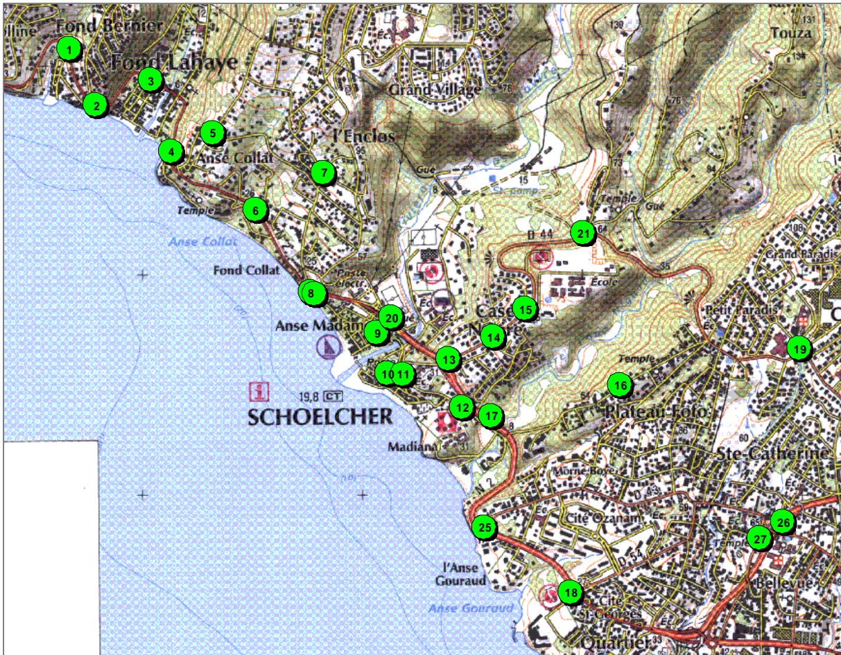
Annexe VI.1 : Implantation des points de mesure sur la commune de Schœlcher.
