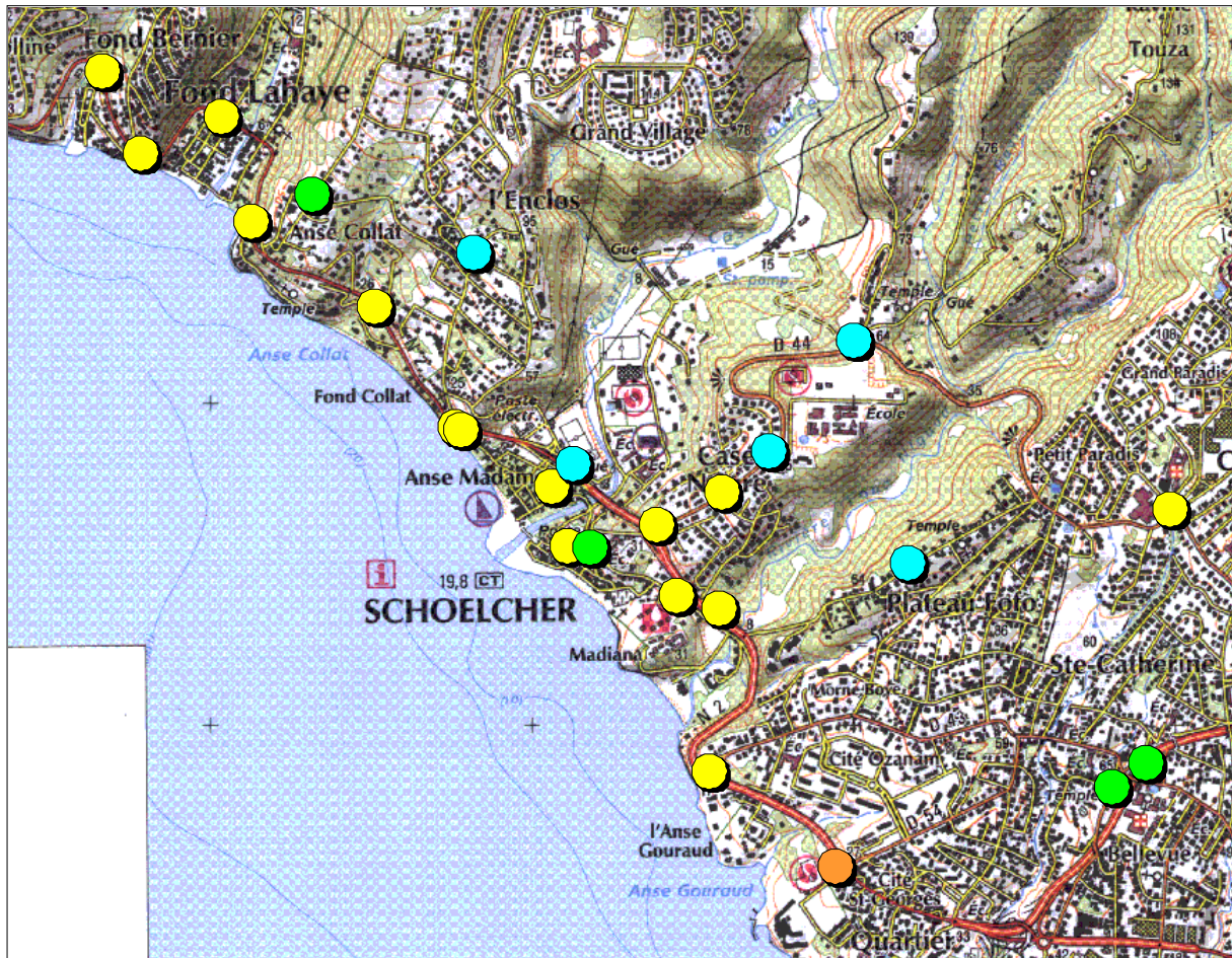
Annexe VI.2 : Dispersion de la concentration en NO 2 ( \mu\text{g}/\text{m}^3 ) sur la commune de Schœlcher durant la Campagne 1 du 15/09/2008 au 29/09/2008.
