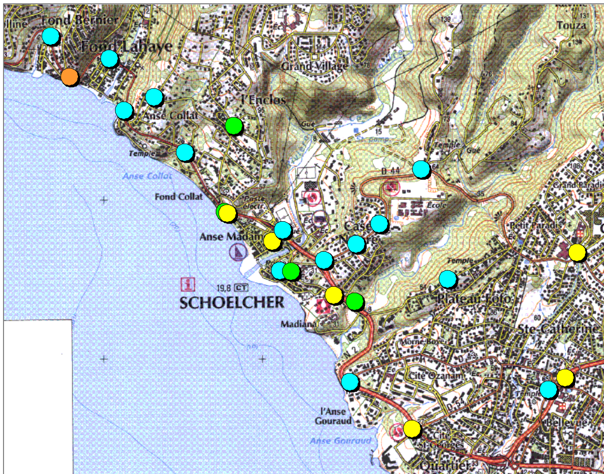
Annexe VI.4 : Dispersion de la concentration en NO 2 ( \mu\text{g}/\text{m}^3 ) sur la commune de Schœlcher durant la Campagne 3 du 03/11/2008 au 17/11/2008.
