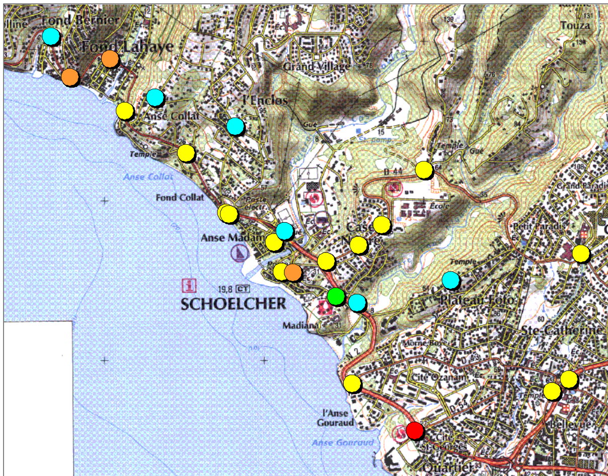
Annexe VI.5 : Dispersion de la concentration en NO 2 ( \mu\text{g}/\text{m}^3 ) sur la commune de Schœlcher durant la Campagne 4 du 17/11/2008 au 01/12/2008.
