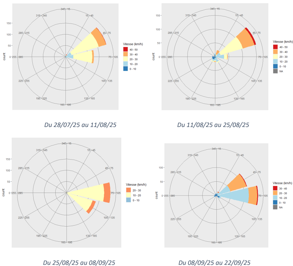
Figure IV-1 : Roses des vents durant la période de mesure sur la station « Robert-Pointe Fort » de Météo France
